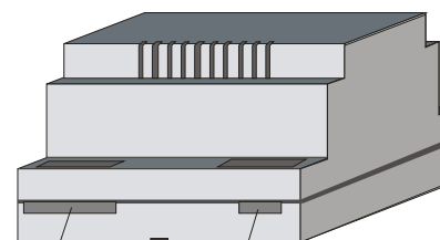
Listwa zaciskowa czujników Gniazdo do podłączenia panelu odczytowo nastawczego
